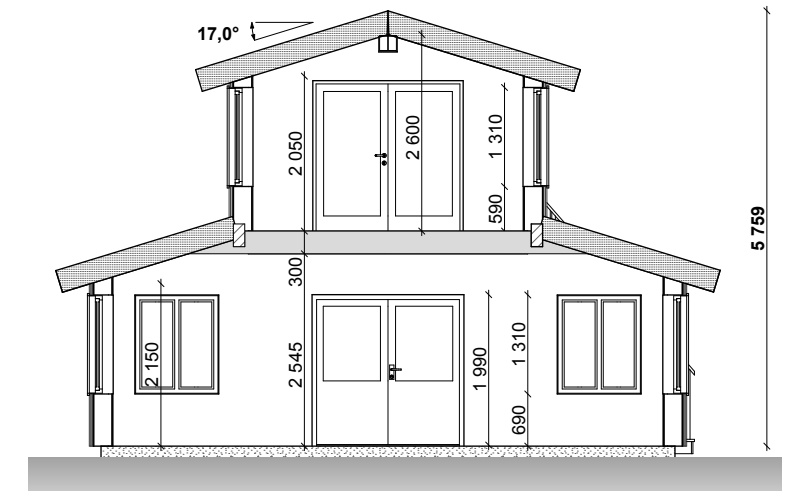
SNITT
