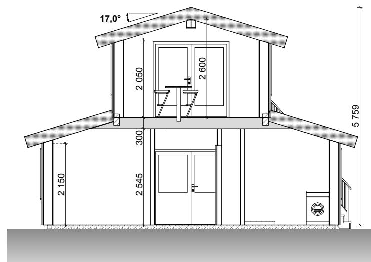
SNITT
